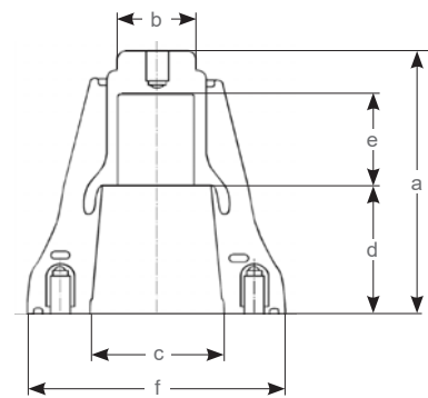
Габаритные размеры Размеры изоляторов RPIS-2-VD и RPIS-3-VD
