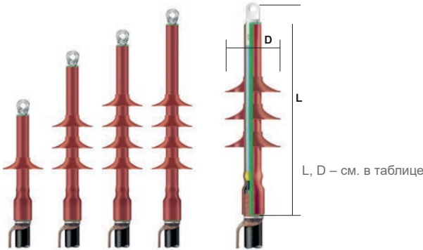
Концевые муфты наружной установки для кабелей с медным проволочным экраном без брони
