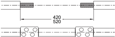
Схема разделки для ремонтной муфты
