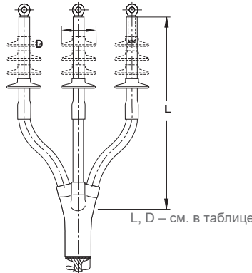
Концевые муфты наружной установки без наконечников и арматуры заземления
