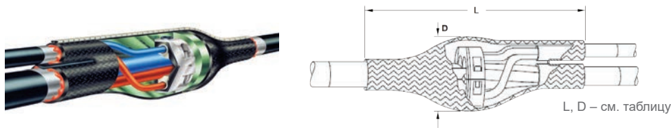
Термоусаживаемые ответвительные муфты для 4-х жильных кабелей с пластмассовой изоляцией в комплекте с изолированным компактным кольцевым соединителем с прокалыванием изоляции
