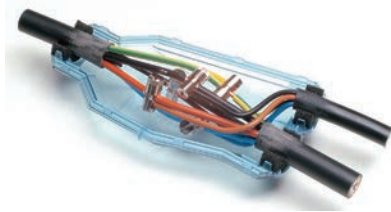
С накидными зажимами
