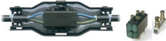
GelBox – соединительные муфты блоком соединителей с прокалыванием изоляцию Максимальное число жил - 4.
