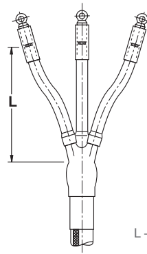
Концевые муфты наружной установки с механическими болтовыми наконечниками и без наконечников
