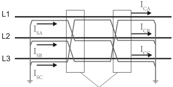
Is- Ток экрана Ic - Ток жилы Муфта или шкаф для транспозиции
