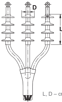
Концевые муфты наружной установки без наконечников и арматуры заземления
