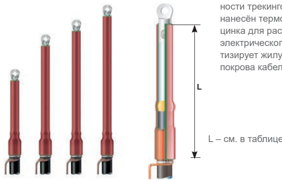
Концевые муфты внутренней установки для кабелей с медным проволочным экраном без брони
