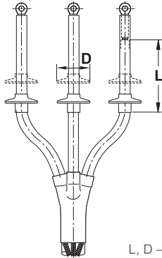
Концевые муфты внутренней установки без наконечников и арматуры заземления
