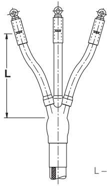
Концевые муфты внутренней установки с механическими болтовыми наконечниками и без наконечников
