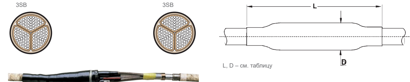
Кабель с общим экраном
