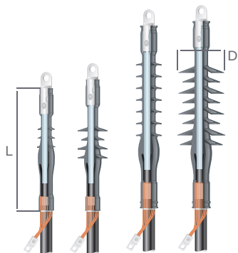
Концевые муфты с механическими болтовыми наконечниками для кабеля с медным проволочным экраном без брони
