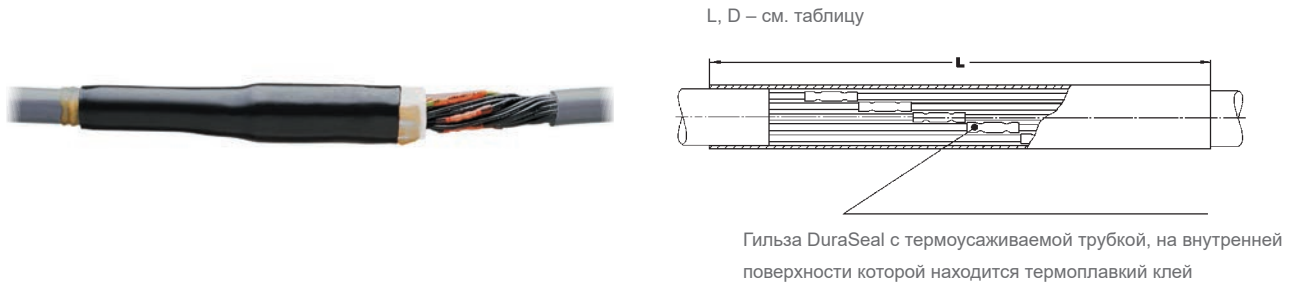
Соединительные муфты для кабелей с пластмассовой изоляцией без брони
