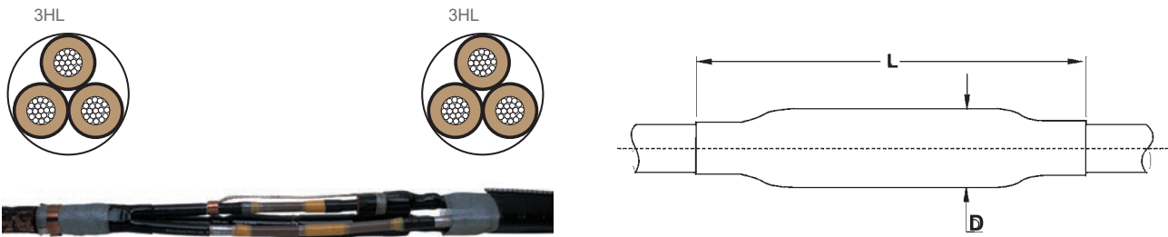
3-х жильный кабель в отдельных оболочках
