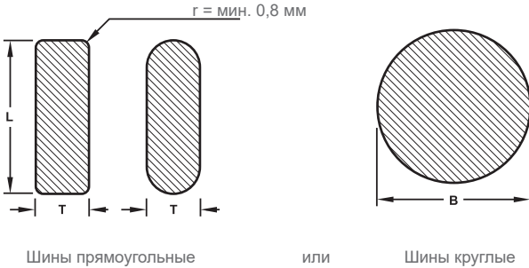
Шины прямоугольные или Шины круглые
